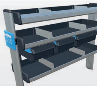
VENSTRE SR5 SMV2 Dim. (BxDxH): 1265x356x1020 mm Vægt: 25,25 kg
