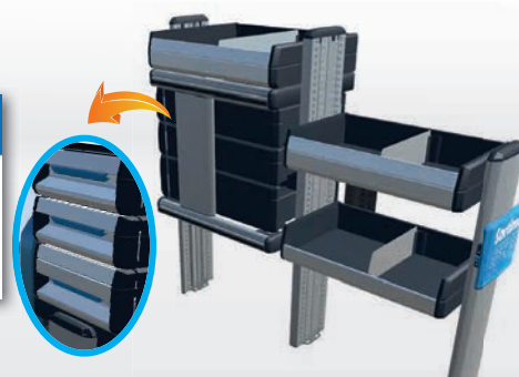
HØJRE SR5 SMH2 Dim. (BxDxH): 1018x356x884 mm Vægt: 37,81 kg
